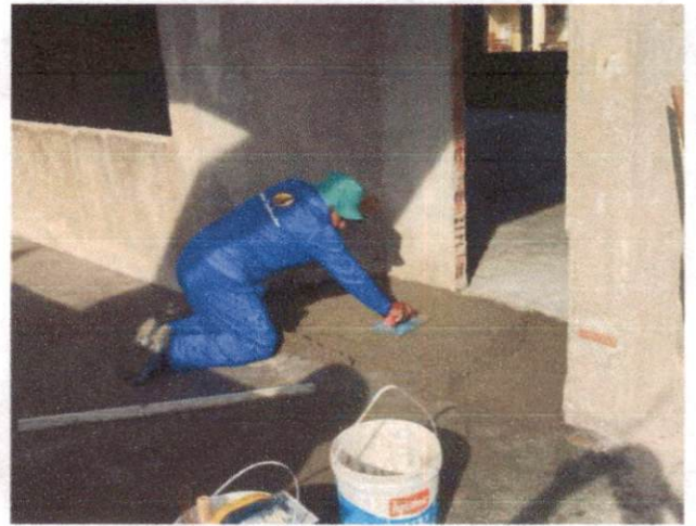
Foto 6: Contrapiso em argamassa traço 1:4 (cimento e areia), aplicado em áreas secas sobre laje, espessura 5 cm. (Item 9.1.2)
